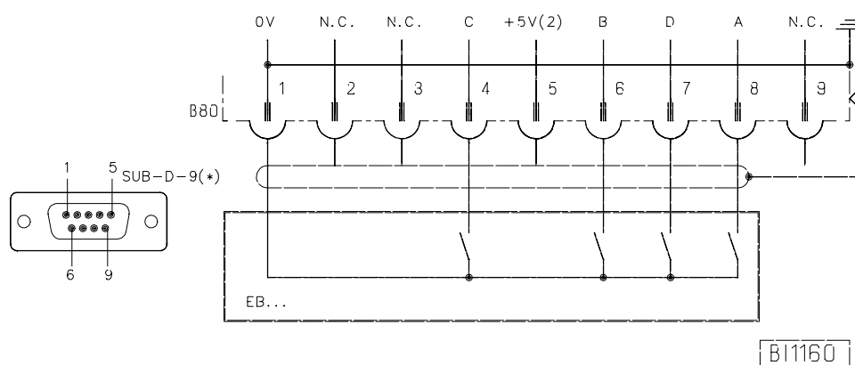
EB.. Actuator
